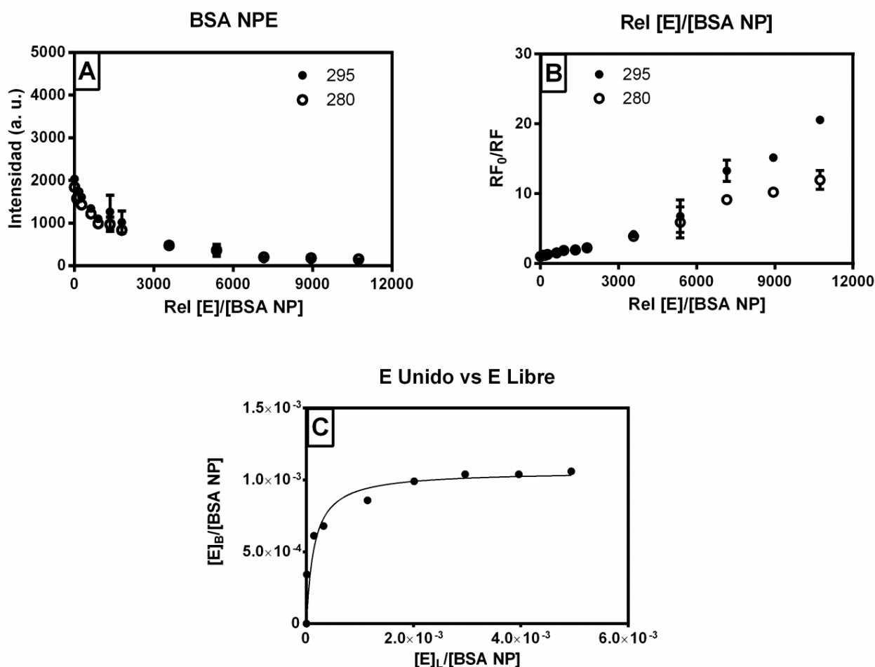
Figura 17 Se representan las curvas de atenuación de la BSA (a) y (c), y de la BSA NP (b) y (d) al interaccionar E con concentraciones crecientes (0.0 – 90.0 μM). Las muestras se excitaron a 280 y 295 nm, con una emisión a 340 y 338 nm, respectivamente. Los datos corresponden a triplicados de las medidas. Representación de las pendientes resultantes de la interacción de E con (a) BSA y (b) BSA NP al excitar las muestras a 280 y 295 nm. Representación gráfica de ajuste usando la ecuación de Scatchard, a partir de la información recolectada según la Figura 35. En este caso, el ajuste se realizó considerando el modelo de regresión no lineal de un sitio de unión (hipérbola) ("One site binding (hyperbola)" from Non-linear regression fit curve).
