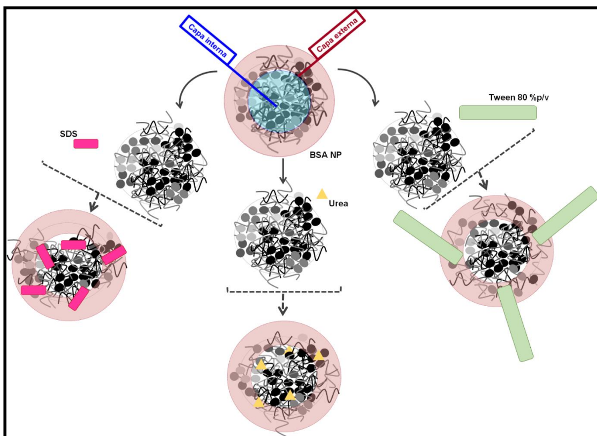
Esquema 12 Ilustración de la BSA NP una vez expuesta a soluciones de Tween 80 %p/v (verde); urea (amarillo) y SDS (rosa). Se centra la atención en el efecto del caotropeo en ambas capas de la BSA NP (interna y externa)
