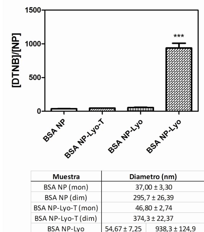
Figura 12 Detección de los tioles libres superficiales en las distintas muestras por medio del método de Ellman. Los resultados obtenidos responden promedios de triplicados de medidas. El análisis estadístico utilizado fue un ANOVA de UNA VIA, P < 0.0001 . Se muestra una tabla con los valores obtenidos, teniendo en cuenta si se trata a la NP como un dímero o monómero de la unidad correspondiente.
