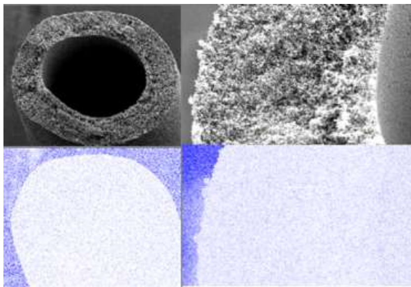
Figura 4.10 – Fotos SEM y \text{Cu}^{2+} -EDAX de corte transversal del material modificado con \text{Cu}^{2+} -IDA. Factor de magnificación 400x y 90x, respectivamente de izquierda a derecha. Visualización de la distribución homogénea del \text{Cu}^{2+} .
