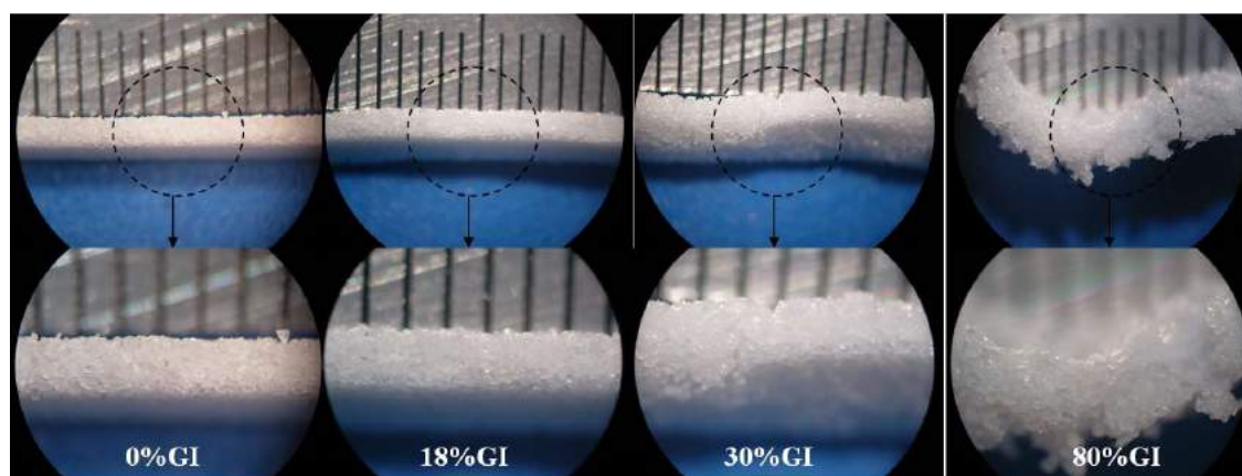
Figura 3.6 – Fotografías de perfil de PE poroso preirradiado en aire y copolimerizado con AAm. De izquierda a derecha: 0 % GI (M2 ó control de copolimerización), 18 % GI (M6), 30 % GI (M5) y 80 % GI (M8). Aumentos en lupa: 1,5x (arriba) y 3x (abajo).
