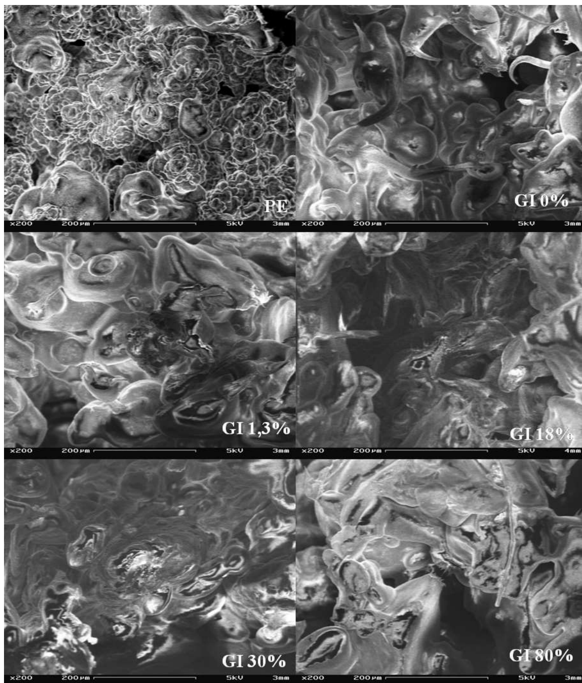
Figura 3.8 – Micrografía SEM. Aumento 200x. Arriba (de izq a der): PE sin irradiar (control sin modificaciones) y PE pre-irradiado con GI 0 % (M2); medio (de izq a der): PE injertado con 1,3 % (M3) y 18 % de AAm (M6); Abajo (de izq a der): 30 %GI (M5) y 80 %GI de AAm (M8).
