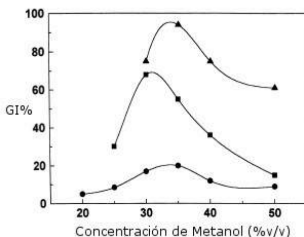
Figura 4.3 – Efecto de la concentración de metanol en el grado de injerto de fibras huecas de PE en soluciones de metanol-agua con 1 % (●), 3 % (■) y 5 % (▲) de GMA. Dosis de radiación: 1,5 kGy (adaptada de Grasselli y col. [6]).
