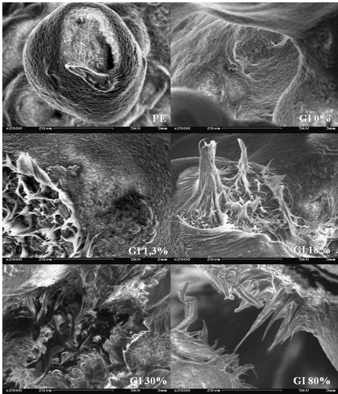
Figura 3.9 – Micrografía SEM. Aumento 2000x. Arriba (de izq. a der.): PE sin irradiar y PE pre-irradiado con GI 0 % (M2); medio (de izq a der): PE injertado con 1,3 % (M3) y 18 % de AAm (M6); Abajo (de izq. a der.): 30 % GI (M5) y 80 % GI de AAm (M8).
