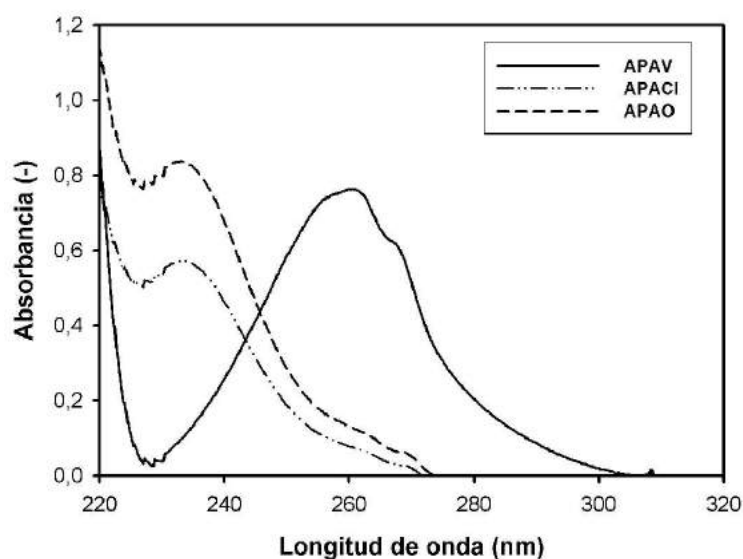
Figura 6.11 – Espectros UV de APAV, APACl (90 % pureza) y APAO (90 % pureza) en HCl 0,1 N.
