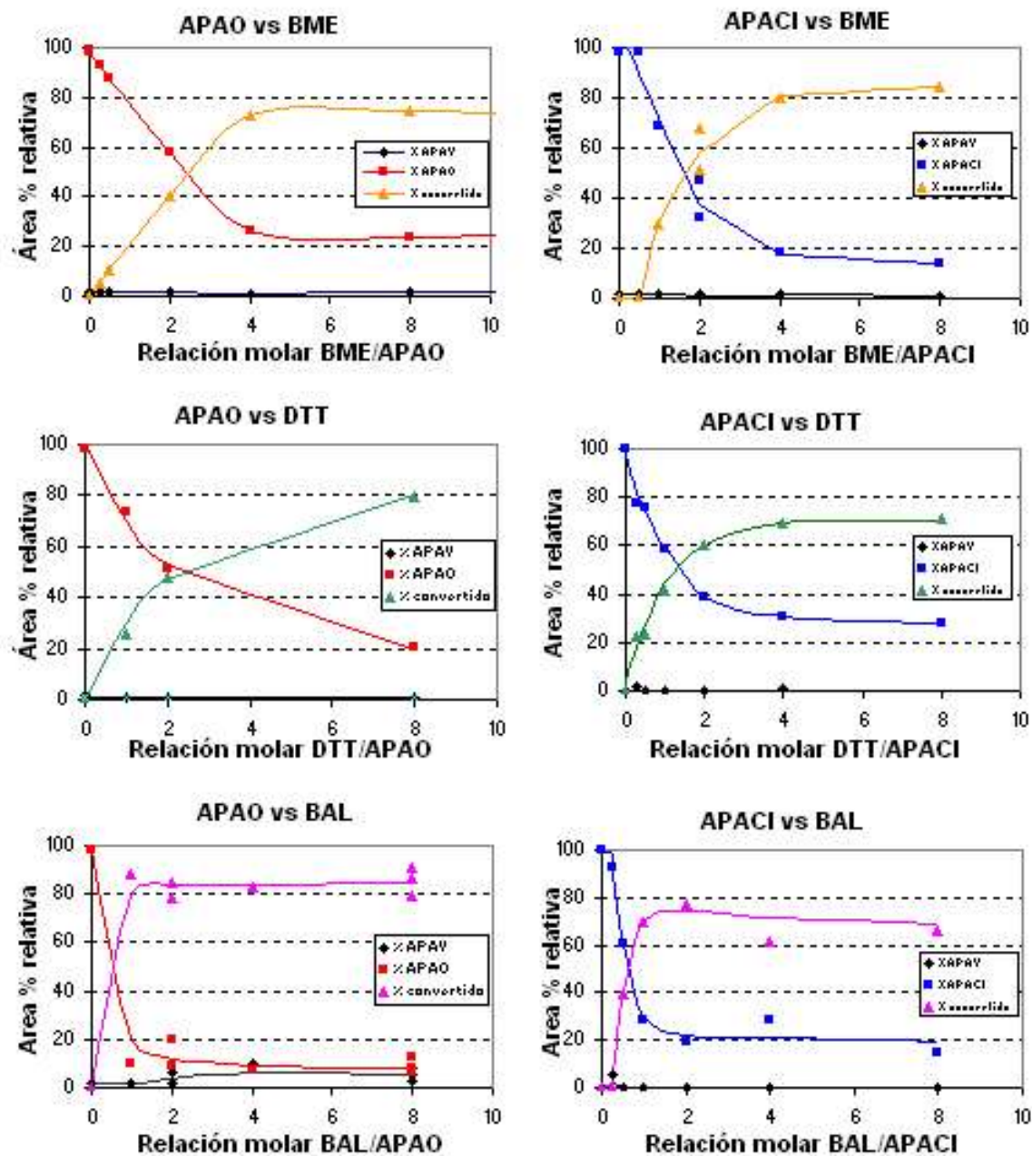
Figura 6.14 – Interacción de los compuestos arseniacales con ditiolos.
