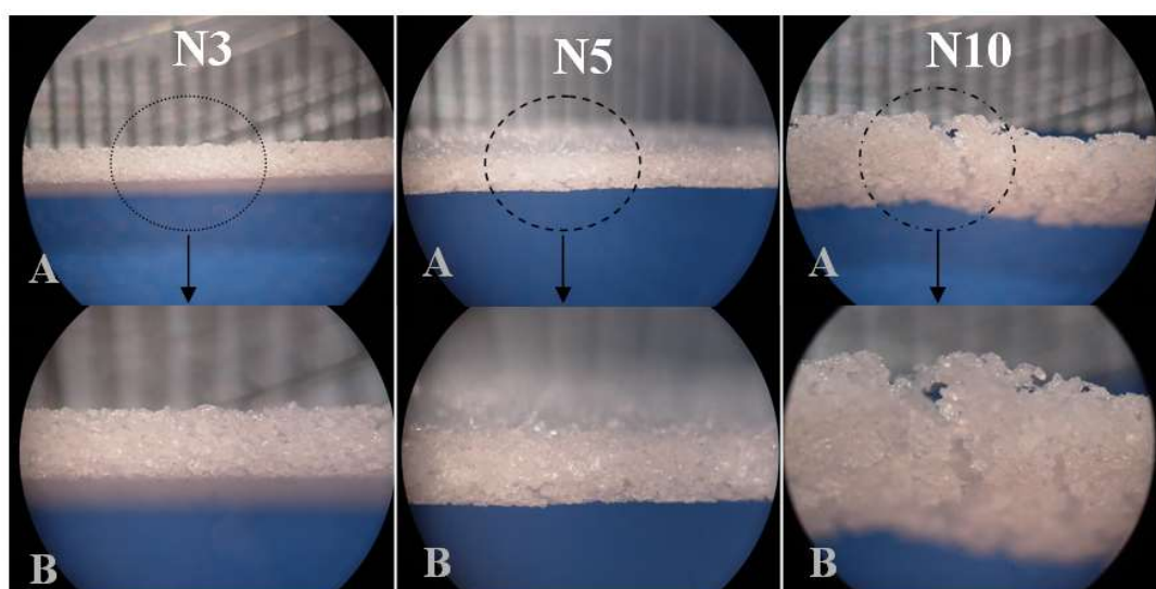
Figura 3.3 – Fotografías ampliadas de perfiles de PE poroso preirradiado en aire y copolimerizado con AAm: N3 (10 % AAm, mezcla etanol agua), N5 (10 % AAm, en agua) y N10 (20 % AAm, en agua). Aumento 1,5x (A) y 3x (B) en lupa. En círculo: zona de A ampliada en B.
