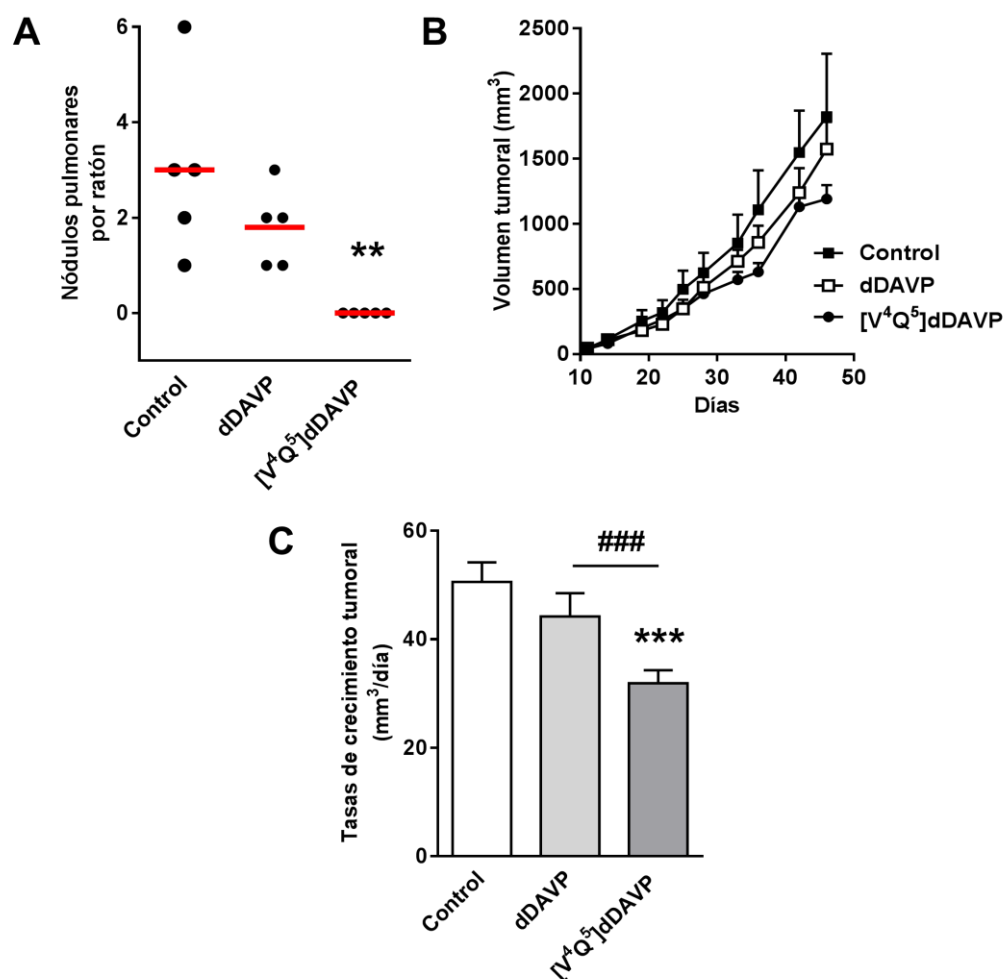
Figura I. 5. Efecto del nuevo análogo [V 4 Q 5 ]dDAVP sobre la progresión tumoral metastásica espontánea en comparación al compuesto parental dDAVP. Para evaluar el efecto sobre la progresión metastásica espontánea de tumores subcutáneos F3II generados en ratones BALB/c, los animales fueron tratados con 3 dosis semanales de 0.3 µg/kg i.v. de dDAVP o [V 4 Q 5 ]dDAVP durante 7 semanas. (A) en el gráfico se observa el número de nódulos pulmonares metastásicos por ratón al finalizar el protocolo. (B) la curva muestra los volúmenes promedio de los tumores F3II creciendo en los flancos subcutáneos de animales pertenecientes a los distintos grupos experimentales. (C) tasas de crecimiento tumoral promedio de los distintos grupos experimentales a partir del día 11 en adelante. Datos expresados como valores ploteados y promedio o promedio ± SD. 5 animales por grupo experimental. **, P<0.01 versus control; ***, P<0.001 versus control, ###, P<0.001 [V 4 Q 5 ]dDAVP versus dDAVP. ANOVA contrastado con Tukey.
