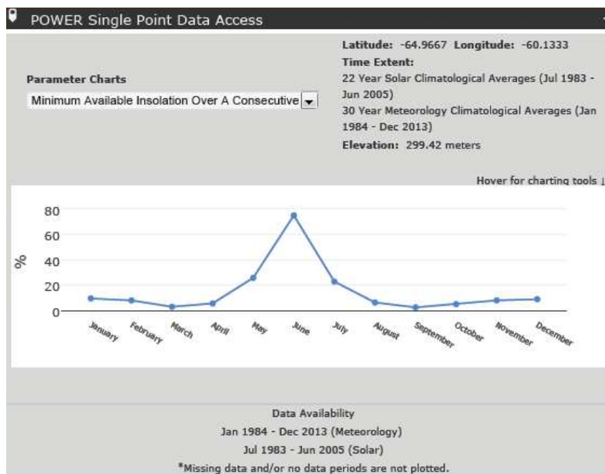
Fig. 40: Valores mínimos promedios de insolación en el período 1983-2005. En el lapso mayo- agosto, con un pico acentuado en el mes de junio, se observa una caída importante de insolación, producto del invierno austral. Fuente: POWER – Data Access Viewer, 2018.
