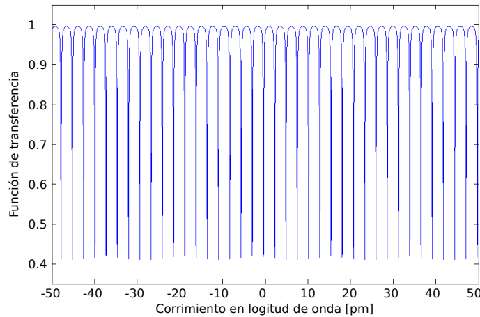
Figura 9.2: Función de transferencia simulada del ARO acoplado al láser DFB en la entrada y considerando una tasa de deriva térmica de 0.2 \text{ nm}/^{\circ}\text{C} . El cambio de temperatura global se ajustó a 0,5^{\circ}\text{C} .
