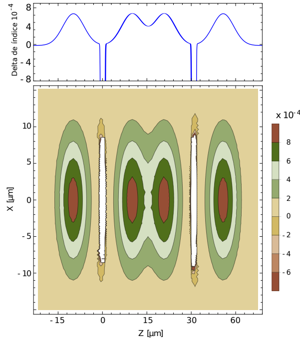
Figura 7.2: Perfil de índice de refracción ordinario y distribución de índice de refracción espacial simulado para parámetros correspondientes a guías de onda escritas dentro de un cristal de \text{LiNbO}_3 según la Ecuación 7.1.
