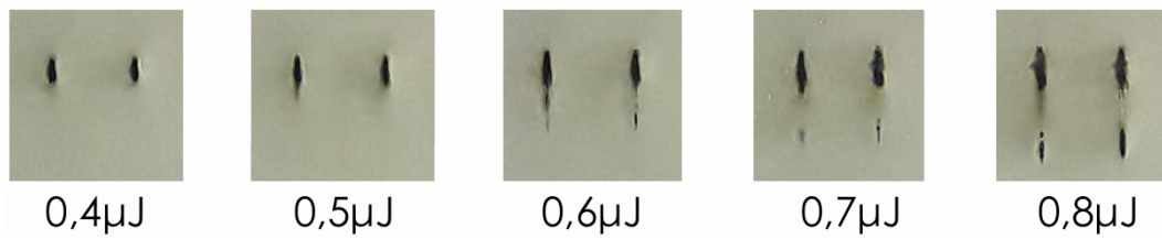
Figura 5.2: Tracks en LiNbO_3 según energía de pulso. A medida que la energía de escritura se incrementa, también aumenta sensiblemente el área de daño en el material.
