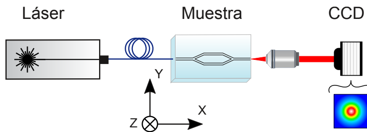
Figura 5.5: Esquema del montaje experimental y acople para caracterizar los modos guiados y las pérdidas de una guía de onda.
