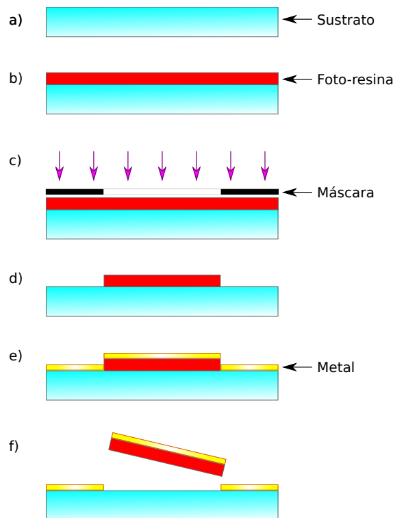
Figura A.1: Proceso litográfico para deposición de electrodos: a) sustrato, b) aplicación de foto-resina, c) curado óptico mediante máscara, revelado de foto-resina, deposición de metal, revelado de metal.
