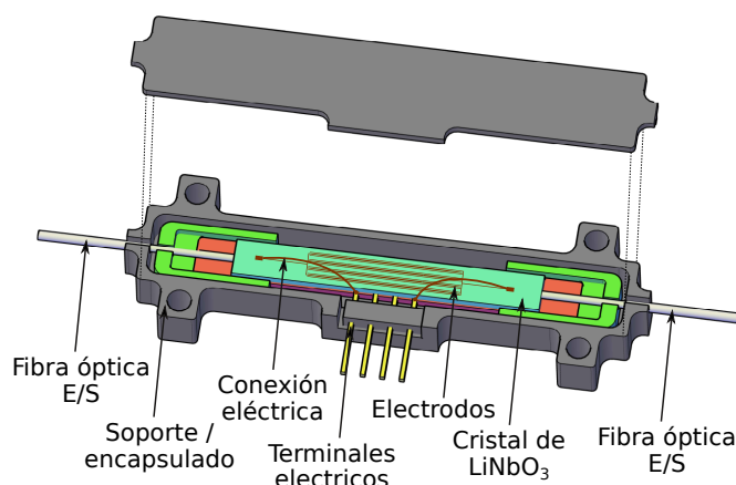
Figura 8.14: Detalle esquemático del IMZ final. Se pueden observar dos canales en los extremos de la caja para alinear las fibras ópticas. La placa de cristal \text{LiNbO}_3 muestra los electrodos depositados y la conexión eléctrica aérea para los terminales de voltaje.
