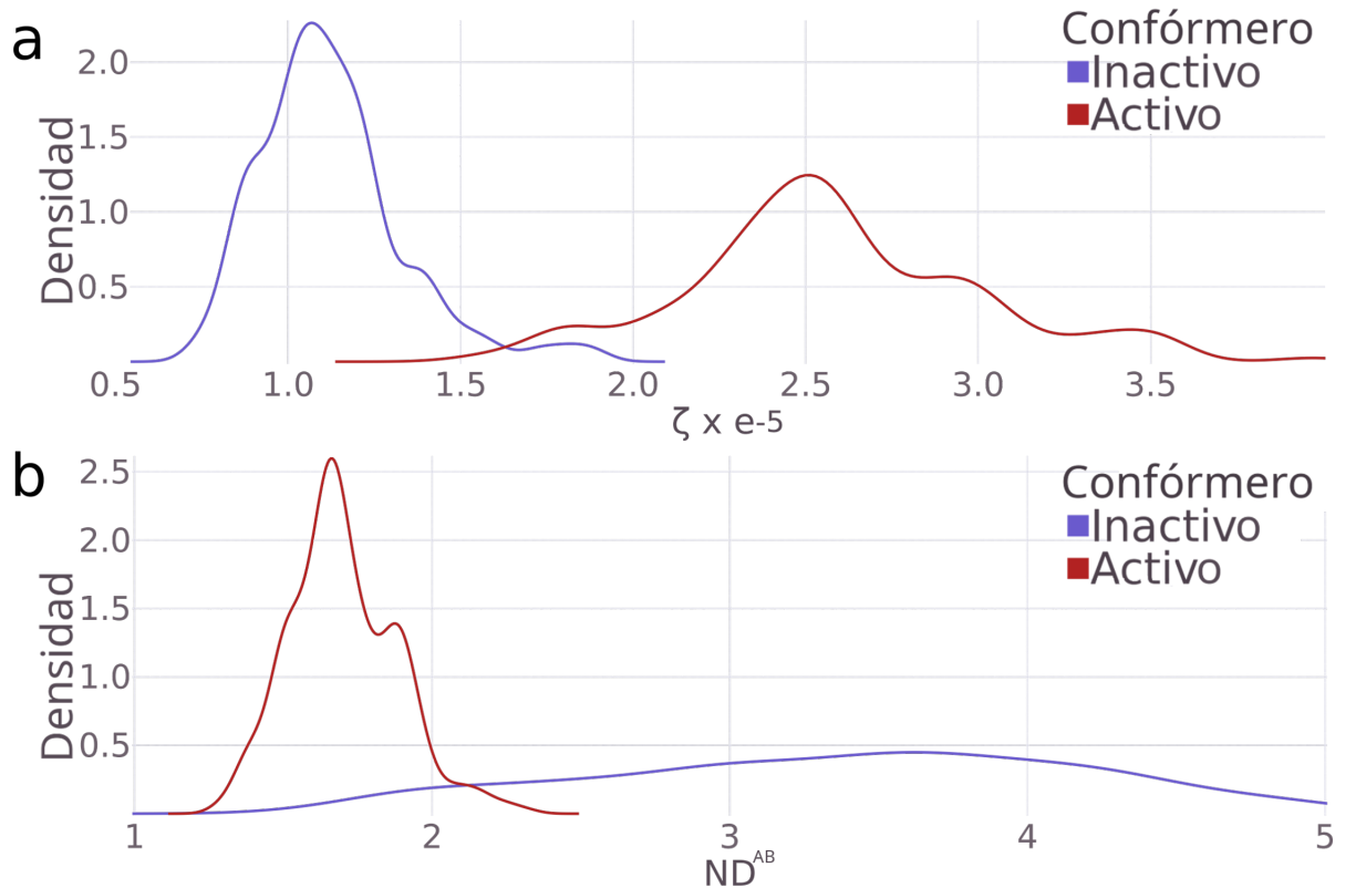
Figure 6.6: Histogramas de valores de a medida de similitud \zeta^{AB} entre pares de subespacios vibracionales ponderados, y b el número efectivo de dimensiones n_D^{AB} compartidas por pares de cónfórmers.
