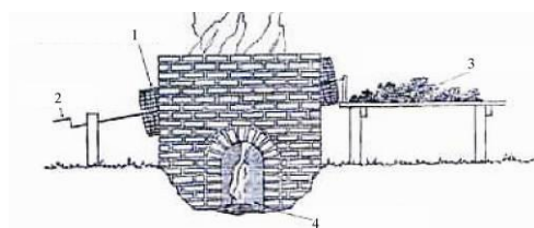
Barbacuá, sapecadora por dentro y su funcionamiento: 1) tambor de alambre tejido; 2) manivela; 3) planchada de hojas verdes; 4) fosa del hornillo. Fuente: www.hohenau.gov.py/detalle.php?idnoticias=52
