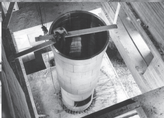
Traslado e instalación del tanque del reactor Fotografías: Archivo CNEA / Gentileza Rafael Castro
