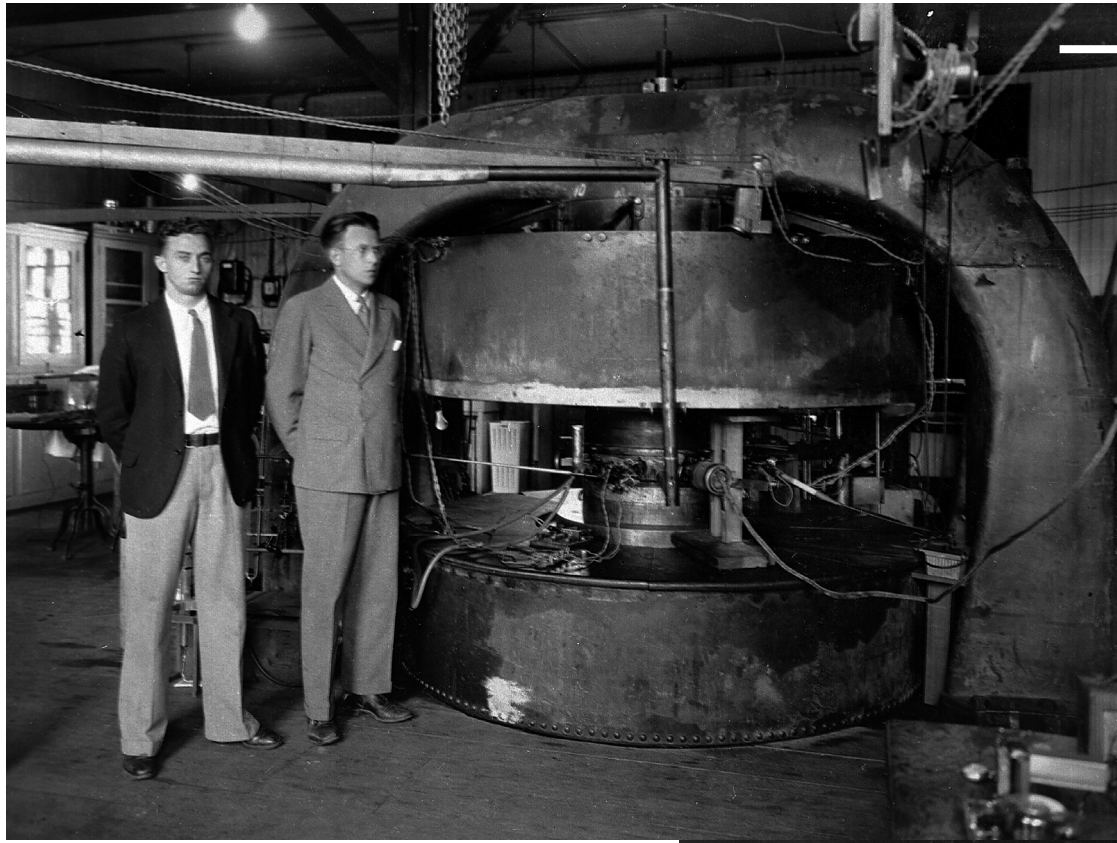
John Lawrence y Stanley Livingston junto las 74 toneladas de hierro y cobre del ciclotrón de 152 cm. (1933)
