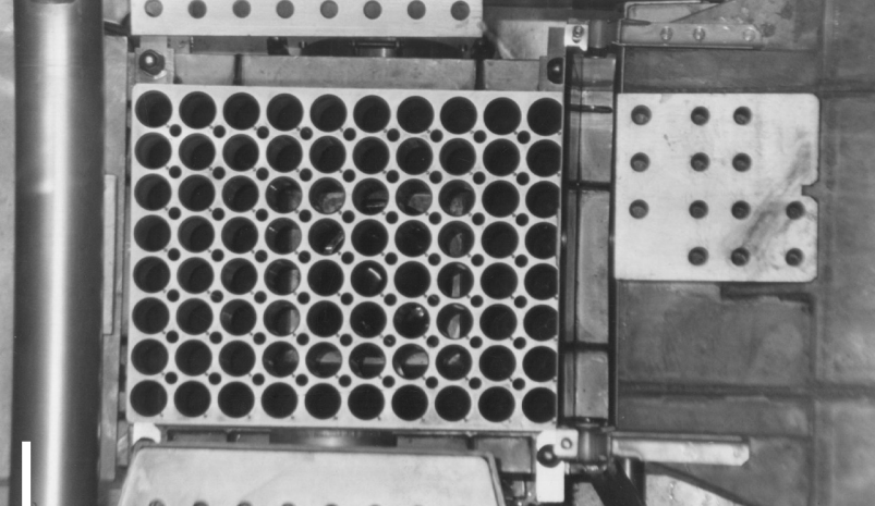
El núcleo del reactor sin los elementos combustibles.
