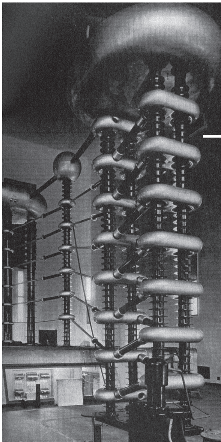
Acelerador en cascada Crockcroft-Walton instalado en 1953 en el patio de la Sede Central de la CNEA.
