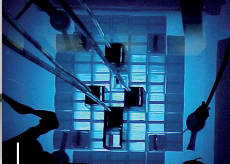
Izquierda: manipulación de las barras de control. Arriba: el núcleo del reactor en funcionamiento.
