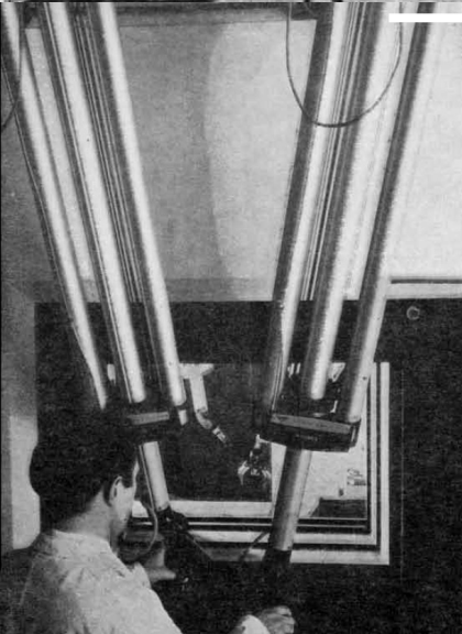
Telemanipuladores de la celda caliente en la planta de Fuentes Intensas. Centro Atómico Ezeiza.
