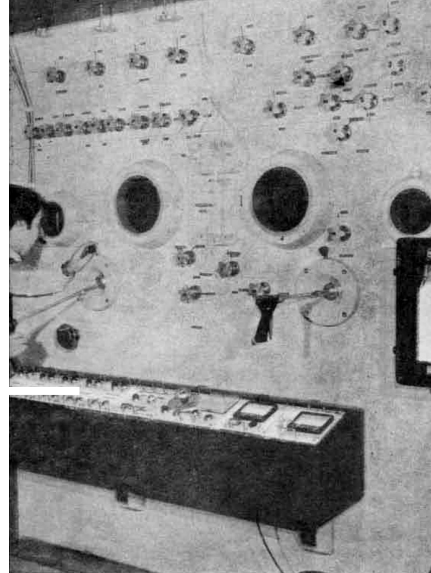
Recinto estanco blindado para la producción de I-131.
