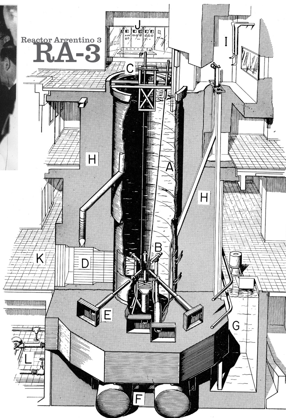
TANQUE DEL REACTOR RA-3 Corte esquemático (CNEA, 1967b)
