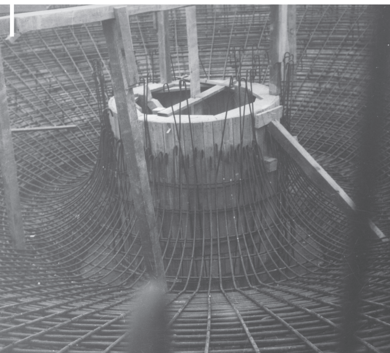
Vistas del avance de la obra civil Fotografías: Archivo CNEA / Gentileza Rafael Castro
