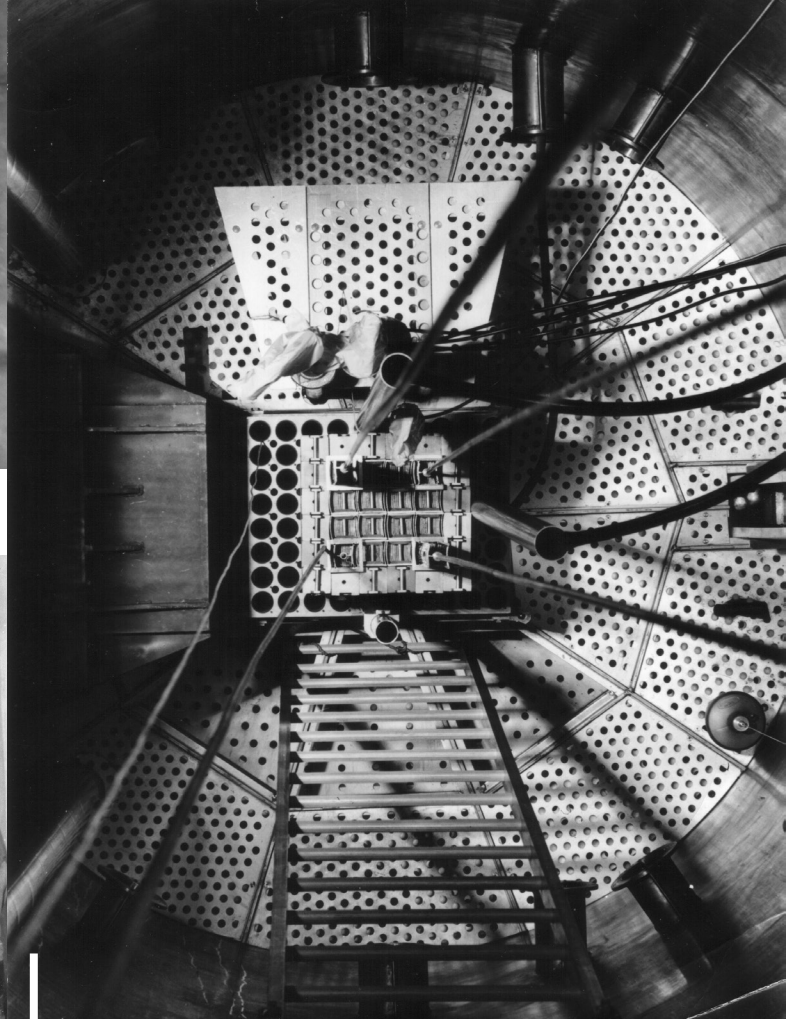
El núcleo del reactor con los elementos combustibles y las barras de control.
