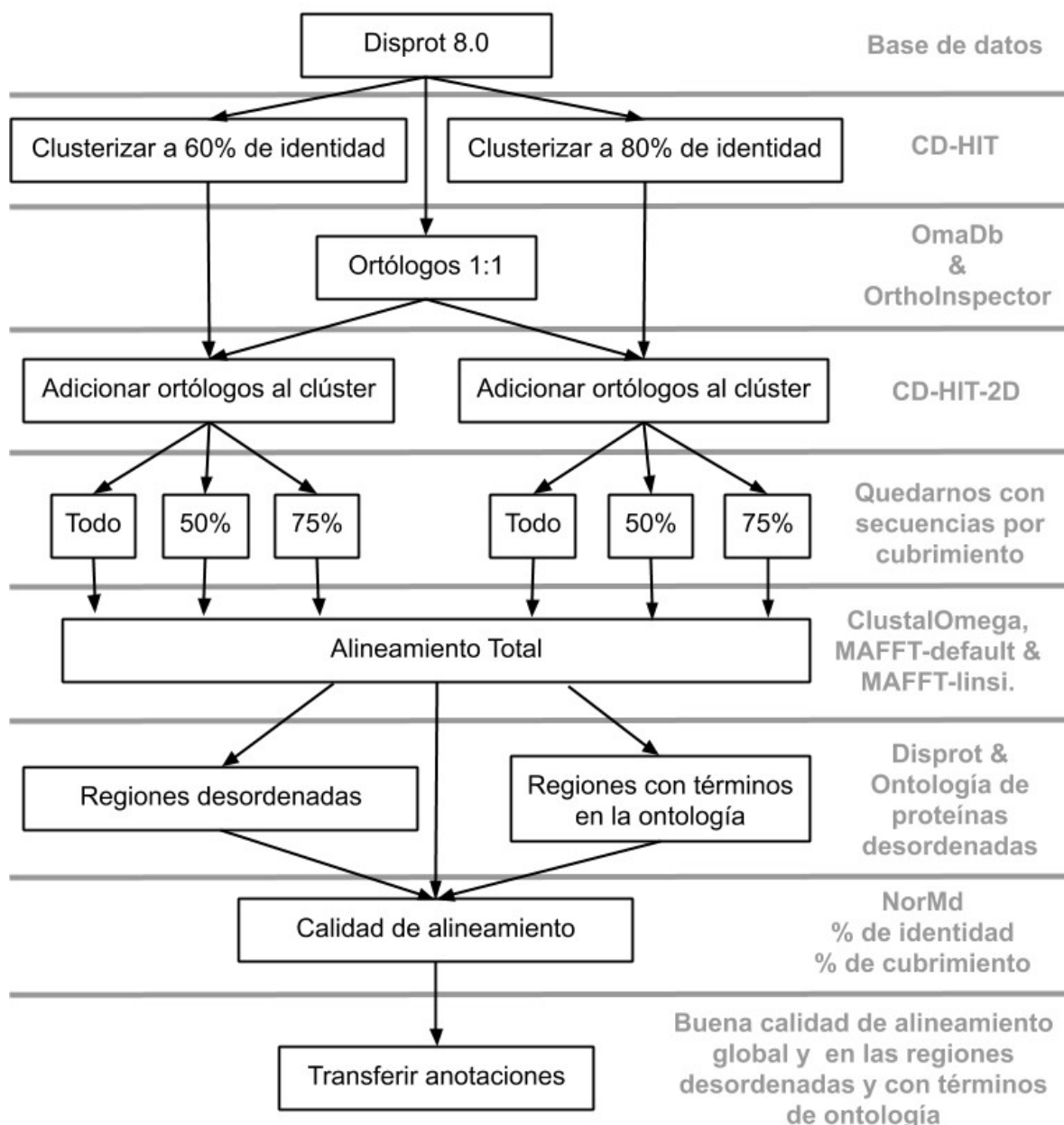
Figura 36. Diagrama general de flujo de trabajo para este proyecto.
