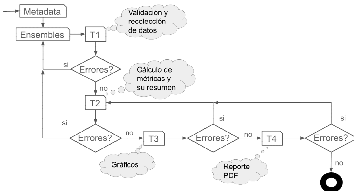
Figura 42. Pipeline utilizado en el servidor para depositar una nueva entrada.
