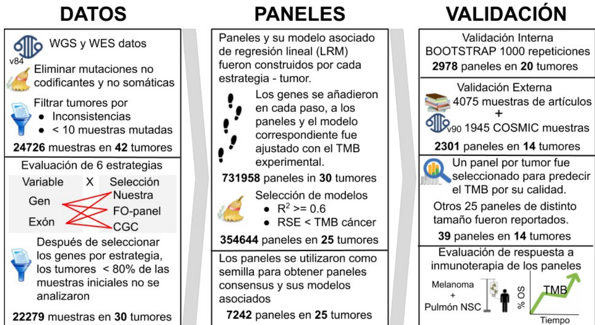
Figura 23. Esquema de trabajo para predicción de TMB.
