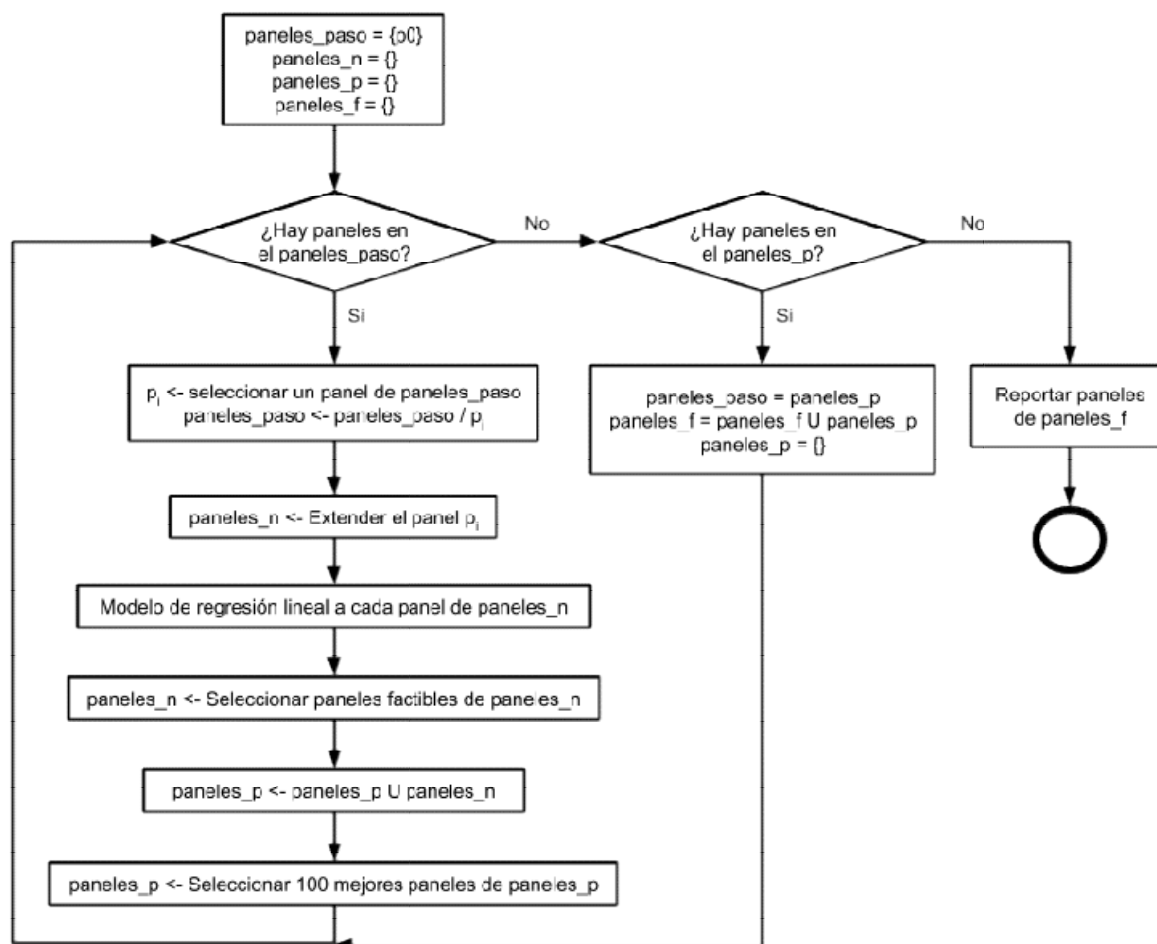
Figura 27. Pseudocódigo del algoritmo ForwardStep utilizado para generar los paneles y modelos de regresión lineal asociados.
