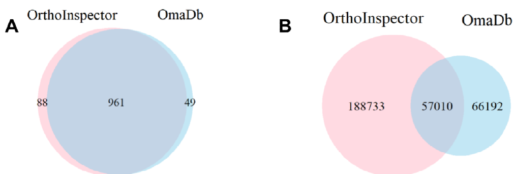
Figura 37. Diagrama de Venn entre las bases de datos de ortólogos.
