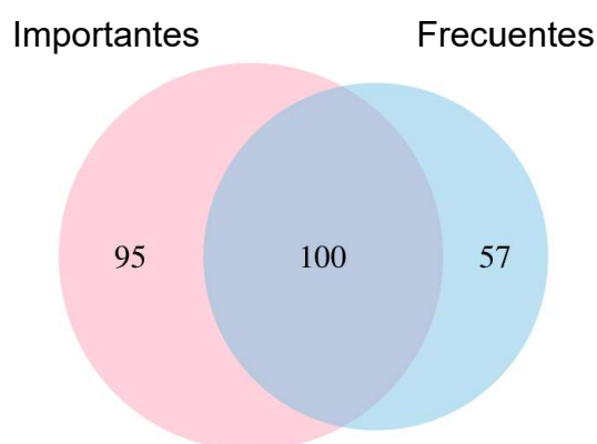
Figura 30. Diagrama de venn entre el top 10 de genes antes y después de la penalización.
