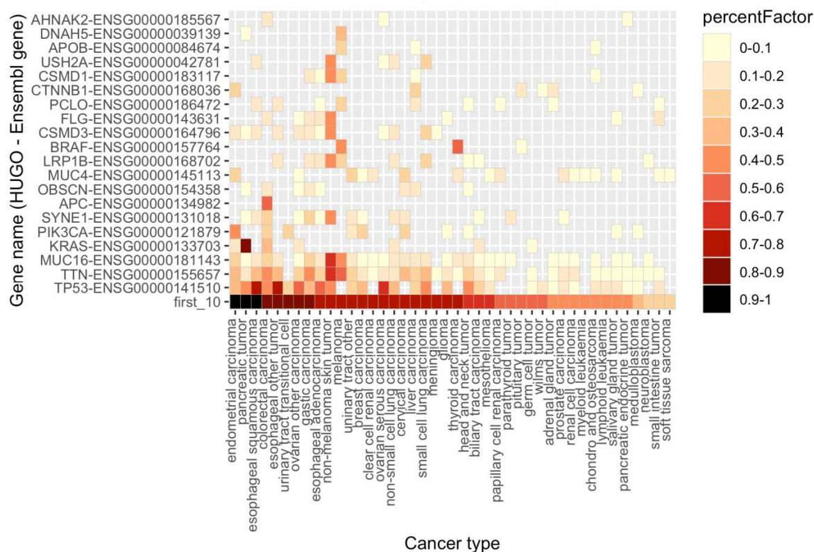
Figura 24. Genes más mutados por tumor.
