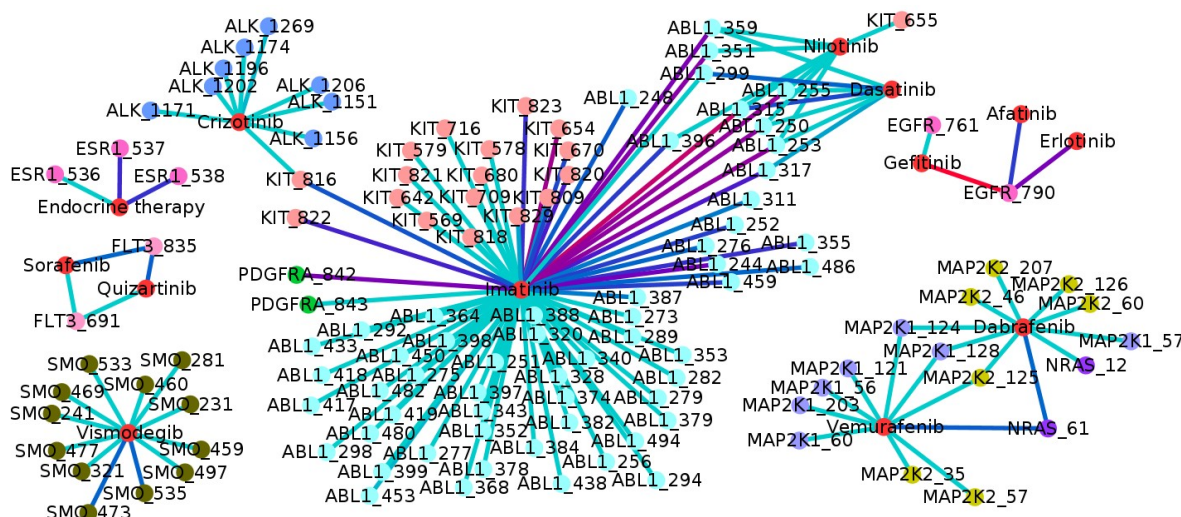
Figura 18. Red de drogas y mutaciones.
