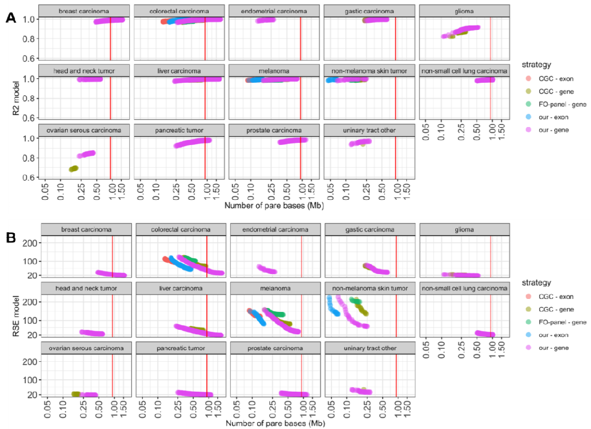
Figura 32. R2 y RSE de los modelos vs longitud en Mb en los 14 tipos de cáncer.
