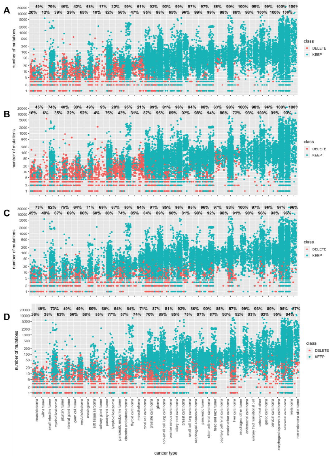
Figura 31. Carga mutacional por tipo de cáncer en las 4 estrategias.
