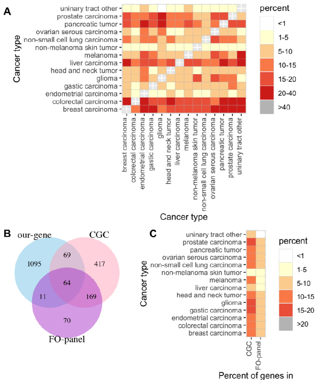
Figura 33. Intersección de los genes presentes en los modelos consensus generados con la estrategia our-gene.
