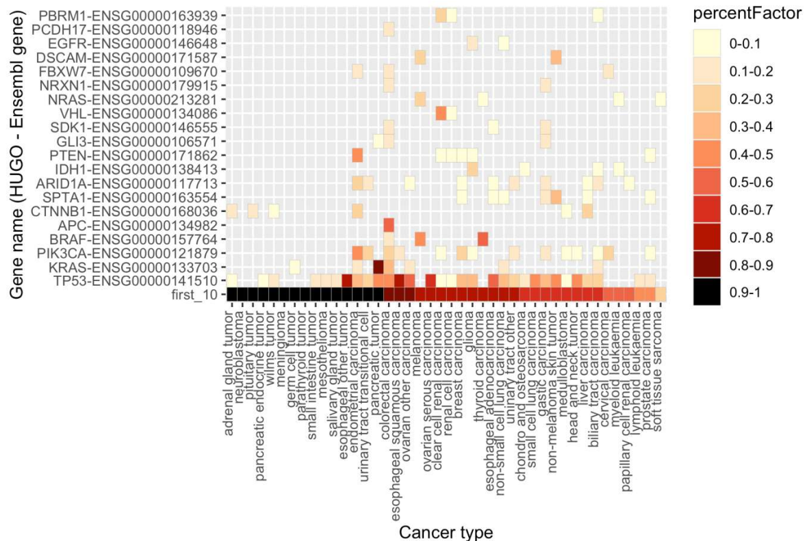
Figura 26. Genes más mutados por tumor después de la penalización por longitud.
