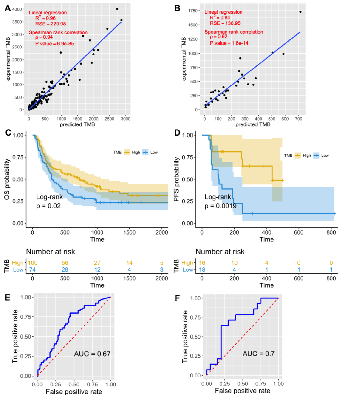
Figura 34. Análisis estadístico relacionado con TMB: la predicción de TMB se realizó con el mejor modelo.
