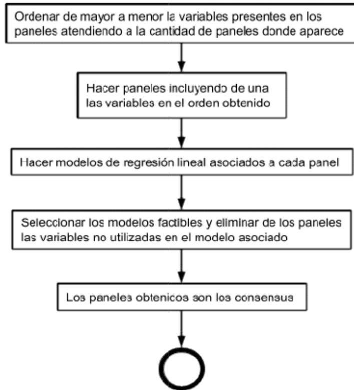
Figura 28. Pseudocódigo para generar los paneles consensus y modelos de regresión lineal asociados.
