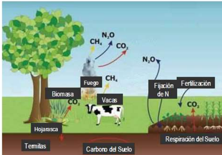
Figura 5. Principales fuentes de emisión de \text{CO}_2 , \text{CH}_4 y \text{N}_2\text{O} provenientes de la agricultura (Modificado de IPCC, 2006).
