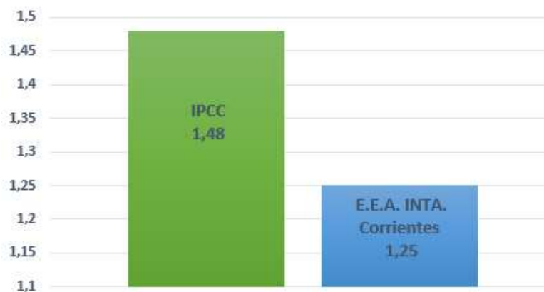
Gráfico comparativo entre factores de emisión de \text{CH}_4 (kg/ha.día)
