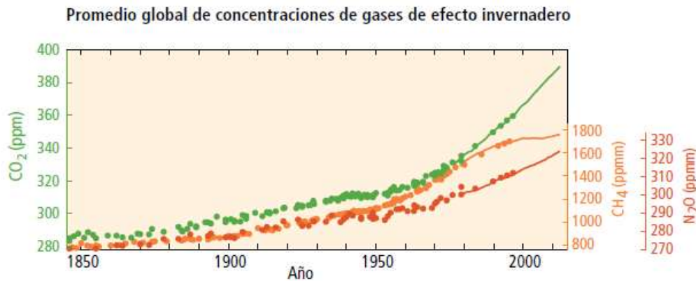
Gráfico 1: Evolución de las concentraciones atmosféricas de gases de efecto invernadero desde mediados del siglo XIX: \text{CO}_2 verde, \text{CH}_4 naranja y \text{N}_2\text{O} rojo; determinados a partir de muestras de hielo (puntos) y de mediciones atmosféricas directas (líneas). Fuente: Quinto Informe del IPCC, 2014.
