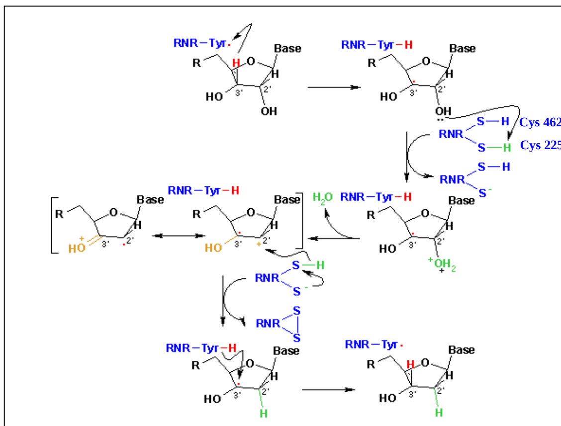
Figura 25: Mecanismo general de reacción de las enzimas ribonucleótido reductasas de clase I.
