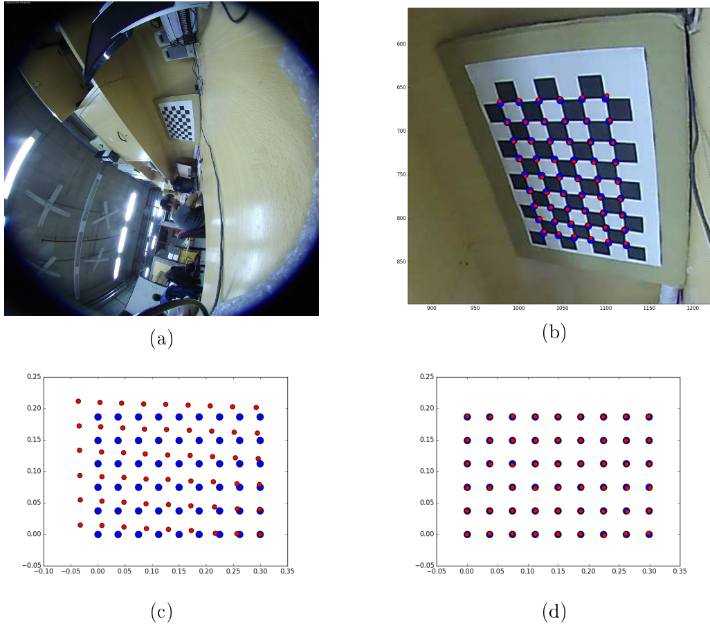
Figura 4.2: (a) Imagen para testear calibración extrínseca. (b) Proyección de puntos de calibración con parámetros que minimizan el error de \mathcal{F} . (c) Retro-Proyección deficiente. (d) Retro-Proyección usando la pose que minimiza el error de \mathcal{G} .
