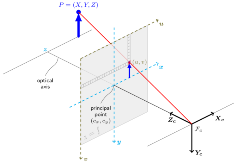
Figura 2.5: Esquema de proyección pinhole de Bradschi [34].
