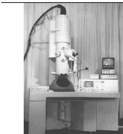
Figura 1. Microscopio electrónico de transmisión PHILIPD CM200 Utratwin, Centro Atómico Bariloche.
