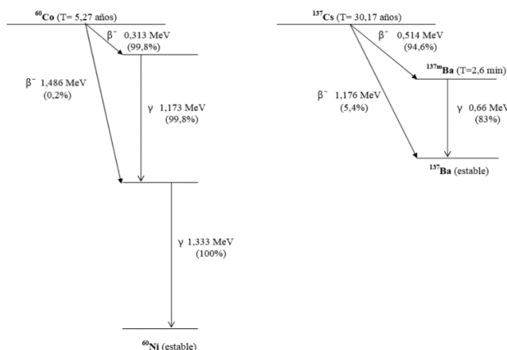
Fig. 7: Esquemas de desintegración simplificados de ^{60}\text{Co} y ^{137}\text{Cs} (IAEA, 2007).
