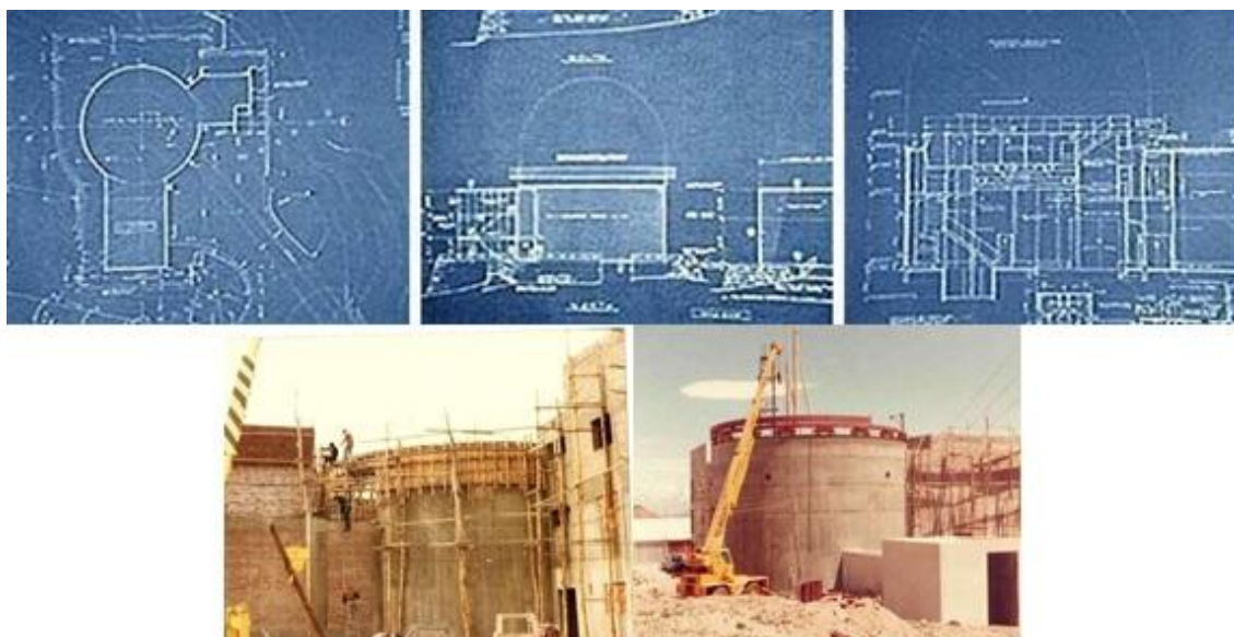
Ilustración 10. Arriba: Detalle de los planos de la cúpula. Abajo: Primeros avances en la construcción de la cúpula. (Fotos de Cristian Willemöes)
