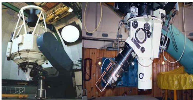
Ilustración 18. Vista del telescopio y del espectrógrafo Echelle de Banco (Fotos de Cristian Willemöes)
