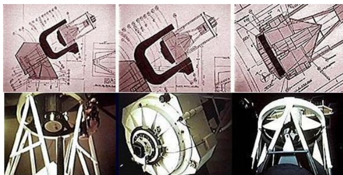
Ilustración 17. Corte de los planos del telescopio platense JS
