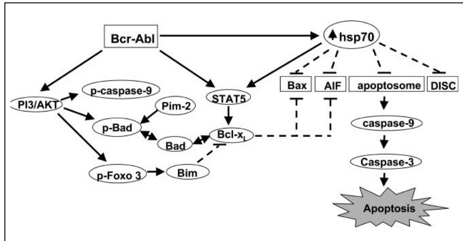
Figura 10. Consecuencia molecular de la sobreexpresión de AKT, STAT5 y HSP70 mediada por BCR-ABL1. La expresión de BCR-ABL1 resulta en una actividad de AKT incrementada (potente mediador de señales antiapoptóticas). AKT fosforila e inactiva BAD, Caspasa-9 y un factor de transcripción Foxo3. Las células leucémicas que expresan BCR-ABL1 también muestran un aumento en la actividad de STAT5, que resulta en un incremento en la expresión de BCL-XL confiriendo resistencia a la apoptosis. Se observa además, un incremento en la actividad de HSP70, que estimula STAT5, además de interferir con la señalización apoptótica en múltiples niveles. (Guo et al , 2005).
