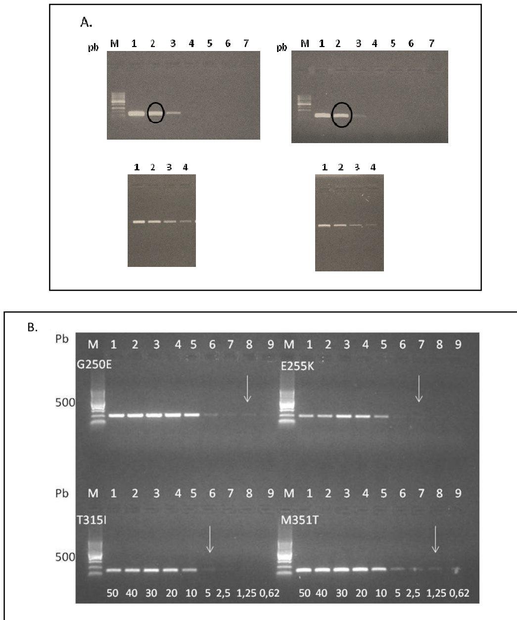
Figura 40. Amplificaciones PCR para determinar el límite de detección de la reacción ASO-PCR. (A). Amplificaciones PCR con primers del Exón3. Panel superior izquierdo: diluciones 10^{-6} - 10^{-12} del plásmido ABL1 Exón6WT-Exón3-Exón4WT. Panel superior derecho: diluciones 10^{-6} - 10^{-12} del plásmido ABL1 Exón6MT-Exón3-Exón4 MT. Panel inferior izquierdo y derecho: amplificaciones PCR comparativas sobre diluciones al medio (1/2, 1/4, 1/8, 1/16) a partir de la primera la dilución donde se observa una clara disminución en la intensidad de señal ( 10^{-7} ). (B). Límite de detección estimado para los ensayos de PCR alelo específica. Las flechas indican la mínima cantidad de alelo mutado reconocido como señal positiva. Para estos experimentos de evaluación de la sensibilidad de cada reacción PCR alelo-específica, se realizaron las mezclas de los constructos ABL1 Exón6MT-Exón3-Exón4 MT en ABL1 Exón6WT-Exón3-Exón4WT (50%; 40%; 30% 20%; 10%; 5%; 2,5%; 1,25%; 0,625%).
