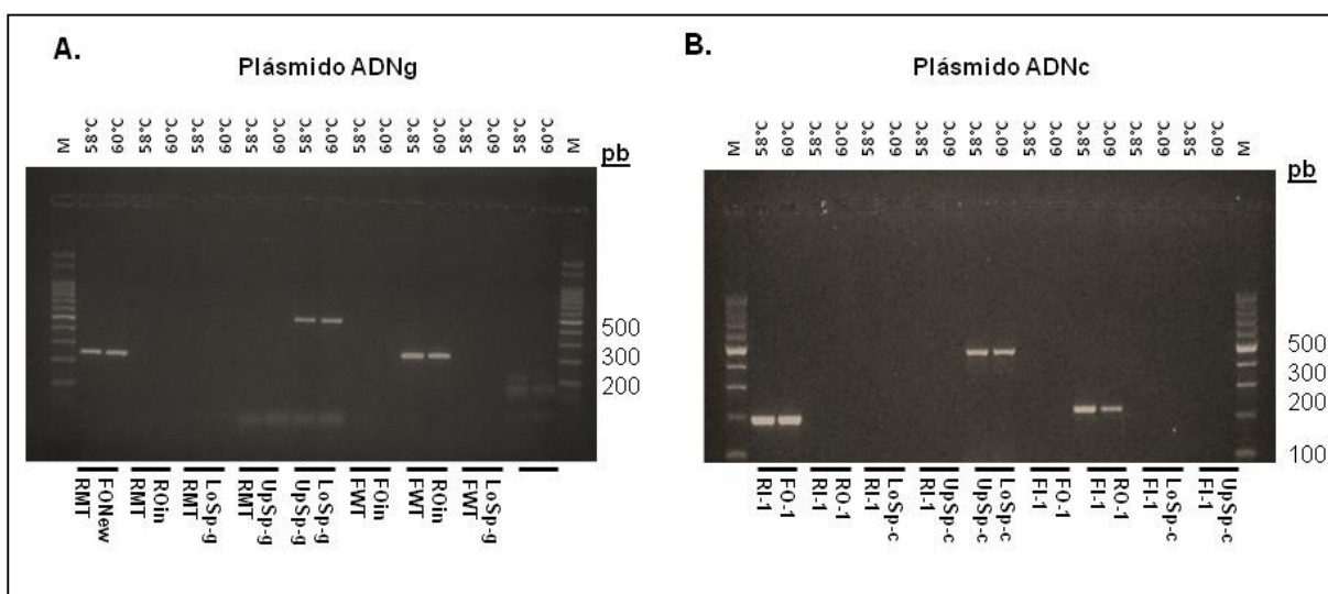
Figura 46. Reactividad cruzada de primers , especificidad estructural de los plásmidos de referencia ADN g y ADN c . Las temperaturas de hibridación y los pares de primers combinados se indican en la parte superior e inferior de la figura respectivamente. Ver Fig 17 y 18 de Material y Métodos para corroborar la especificidad de los primers para generar productos PCR sobre los constructos de ADN g (A) y ADN c (B).
