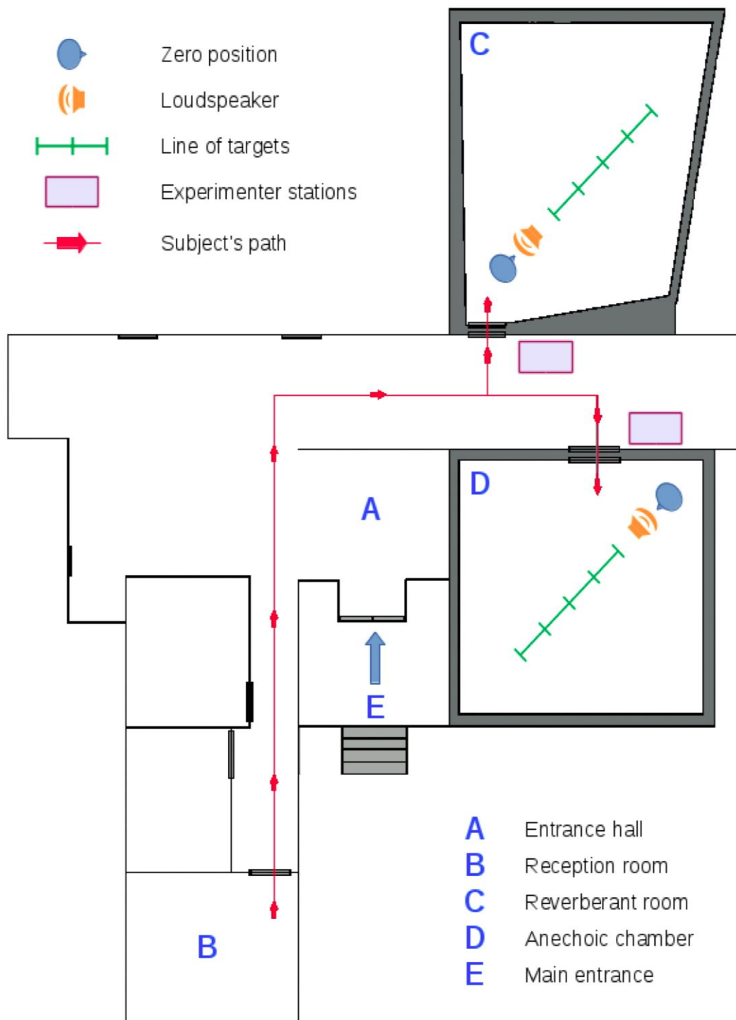
Figura 9.1: Diagrama de la instalación experimental en el Laboratorio de Acústica y Luminotecnia. Se observa la habitación reverberante (C), la cámara anecoica (D), el camino recorrido por los sujetos (con los ojos cubiertos) durante los experimentos desde que fueron recibidos (A) a la sala de recepción (B, donde fueron informados). Ya ambas salas de pruebas
