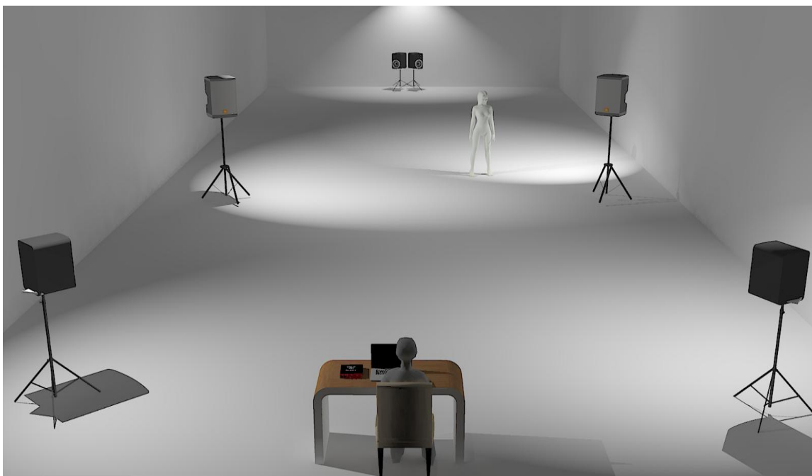
Figura 10.10: Esquema de la disposición de parlantes para la obra escénica LEJOS . Dos cajas de mayores dimensiones, ubicadas a ambos lados del escenario (PA), dos cajas de menores dimensiones ubicadas detrás de la platea y dos cajas juntas ubicadas detrás de la escenografía.
