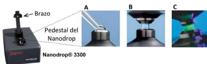
Fig.2.6. Esquema del procedimiento estándar de medida del equipo (muestras líquidas). A- Siembra de la muestra sobre el pedestal. B- Apoyo del brazo sobre el pedestal, toma de medida y formación de la columna de líquido de 1 mm de alto. C- Excitación de la muestra con la longitud de onda correspondiente y cuantificación de la emisión de fluorescencia.
