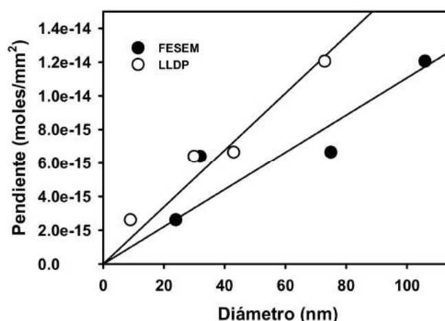
Fig. 2.23. Pendiente de CTM con Fluoresceína en función del diámetro determinado por la técnica de ● FESEM y ○ LLDP.
