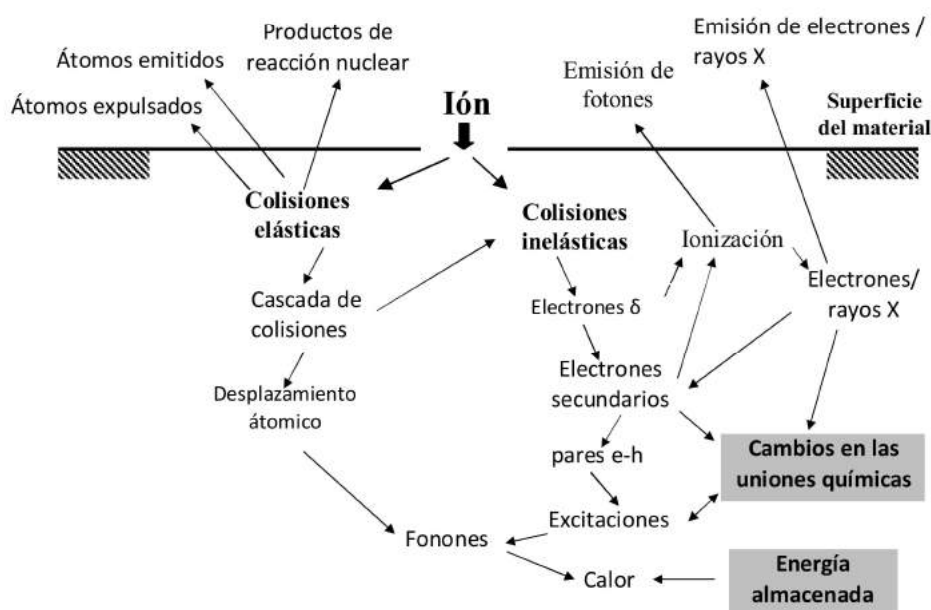
Fig. 1.9. Procesos físico-químicos que ocurren en un material irradiado con iones acelerados.
