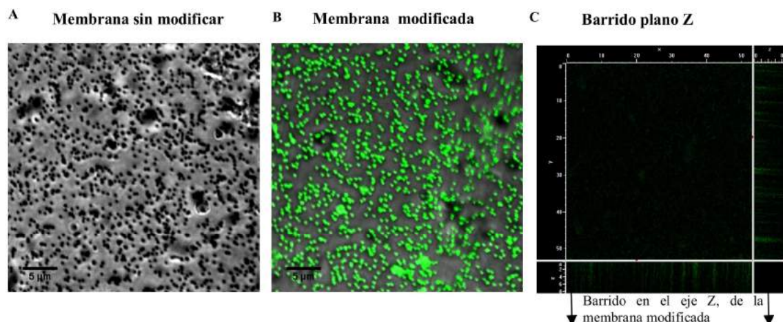
Fig.3.15. Imágenes de microscopía de fluorescencia, con un zoom de imagen de 4x (magnificación total 240x). A Membrana sin modificar. B. Membrana modificada y derivatizada. C. Microscopía Confocal de barrido en el eje Z, se tomaron secciones cada 0,25 µm (distancia en el eje Z= 8 µm).
