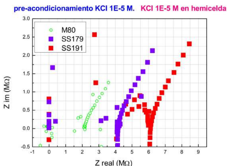
Fig. 2.31. Gráfico de Nyquist correspondiente a las mediciones de EIS de membranas pre-acondicionada con KCl 1\text{E}-5 M. PET SS179 (cuadrado violeta ■), SS191 (cuadrado rojo ■) y PC M80 (círculo vacío ○).
