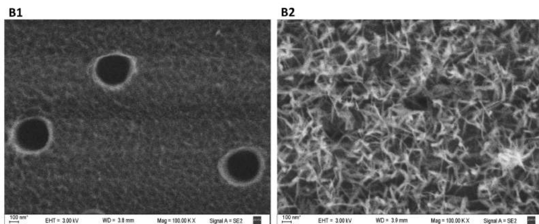
Fig.3.5. Micrografías de membranas PET modificadas por la técnica PIVRR-C/SM . A-1. Membrana SS34. A-2. Membrana SS34 modificada, 1h. B-1. Membrana SS17. B-2. Membrana SS17 modificada, O.N.
