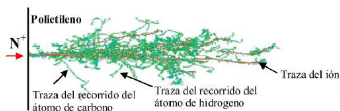
Fig. 1.12. Resultado del cálculo mediante el código TRIM, para la penetración de 10 iones de Nitrógeno a 20 keV, en PE.
