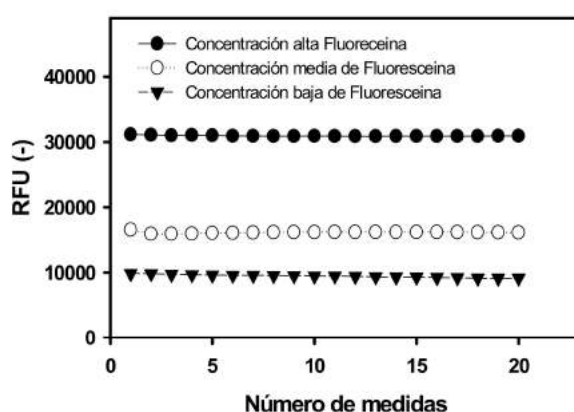
Fig. 2.19. Ensayo de Blanqueamiento, para tres soluciones de fluoresceína. ● 0,7 \mu\text{M} . ○ 0,37 \mu\text{M} . ▼ 0,22 \mu\text{M} .
