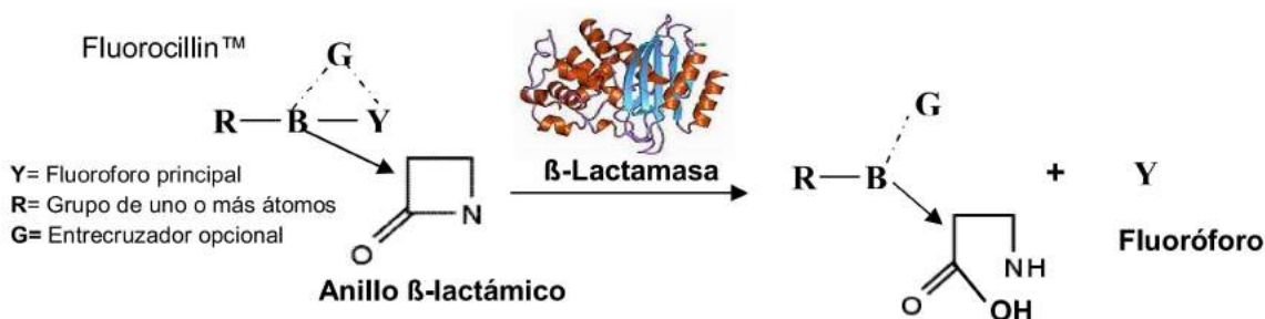
Fig.5.1. Esquema de la acción hidrolítica de la β-Lactamasa sobre el Fluorocillin™.
